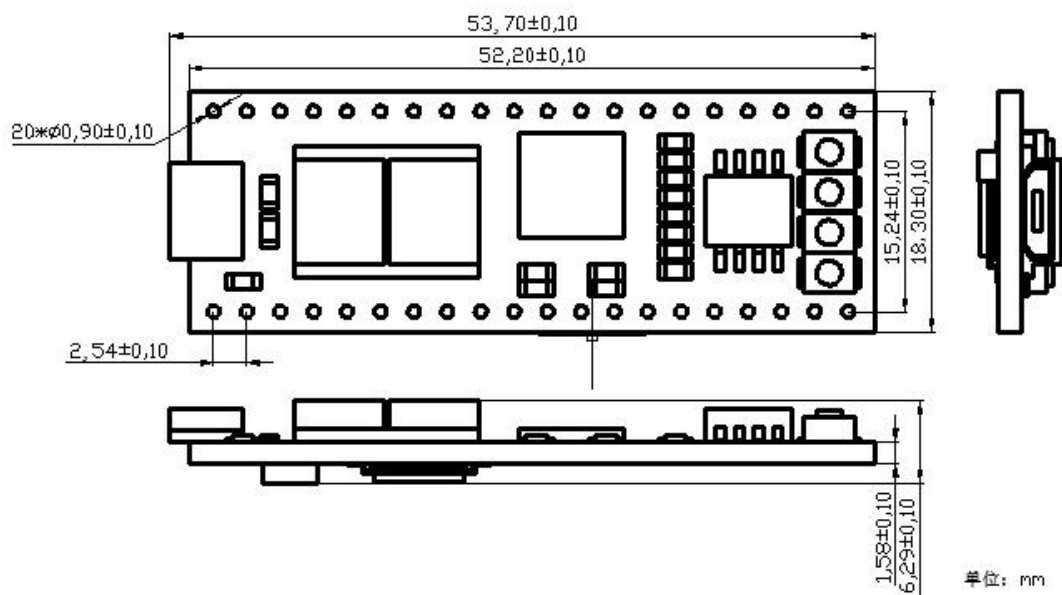
图 6 STEP MX02 结构图
